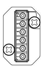
モータ側コネクタ結線仕様
